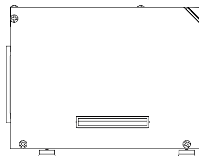
ZIJAANZICHT (L)
